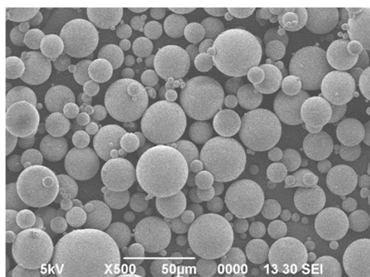
SEM画像
