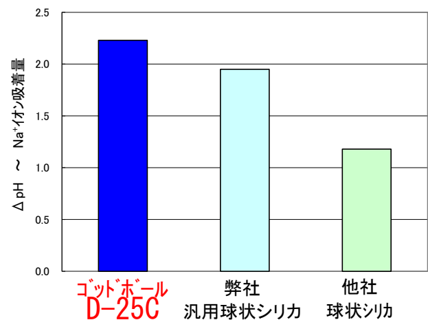
Na + イオン吸着試験結果(ΔpH測定*)
